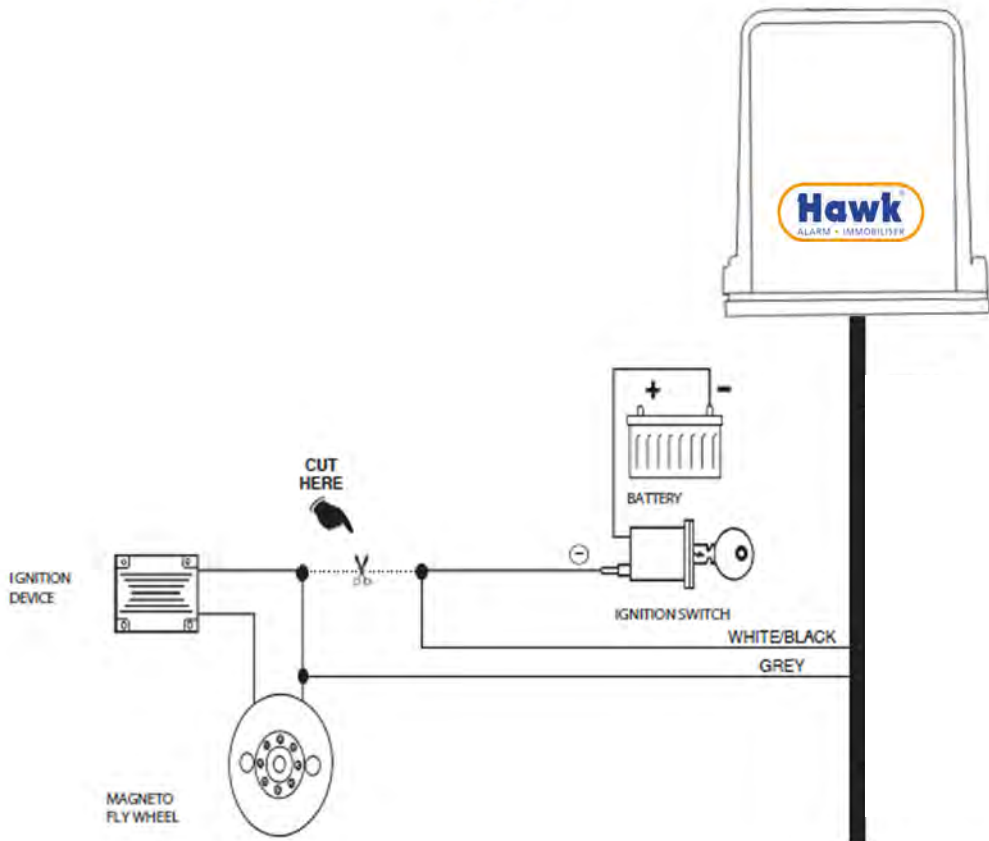
Fig. 2 (AC)
