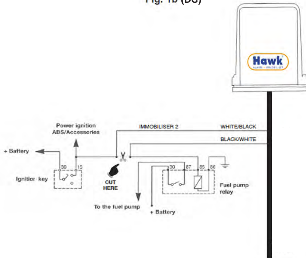
Fig. 1b (DC)
